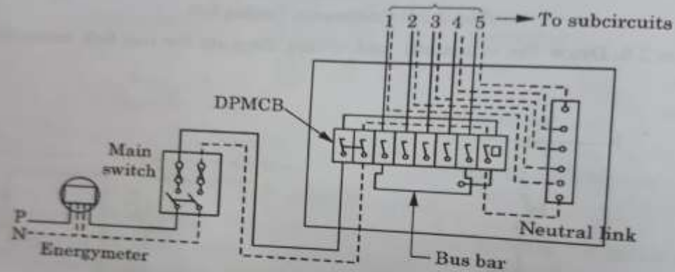
Fig. 2.29: Wiring diagram
