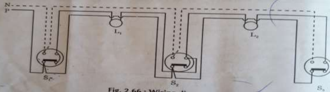
Fig. 2.66 : Wiring diagram
