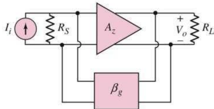
(d) Shunt-shunt
